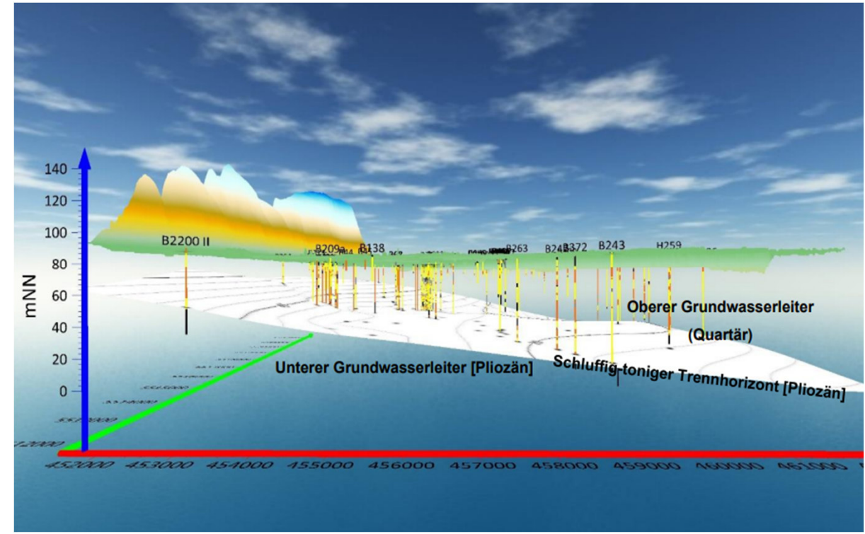
Abb. 4: Geosystemanalyse Guntersblum.
