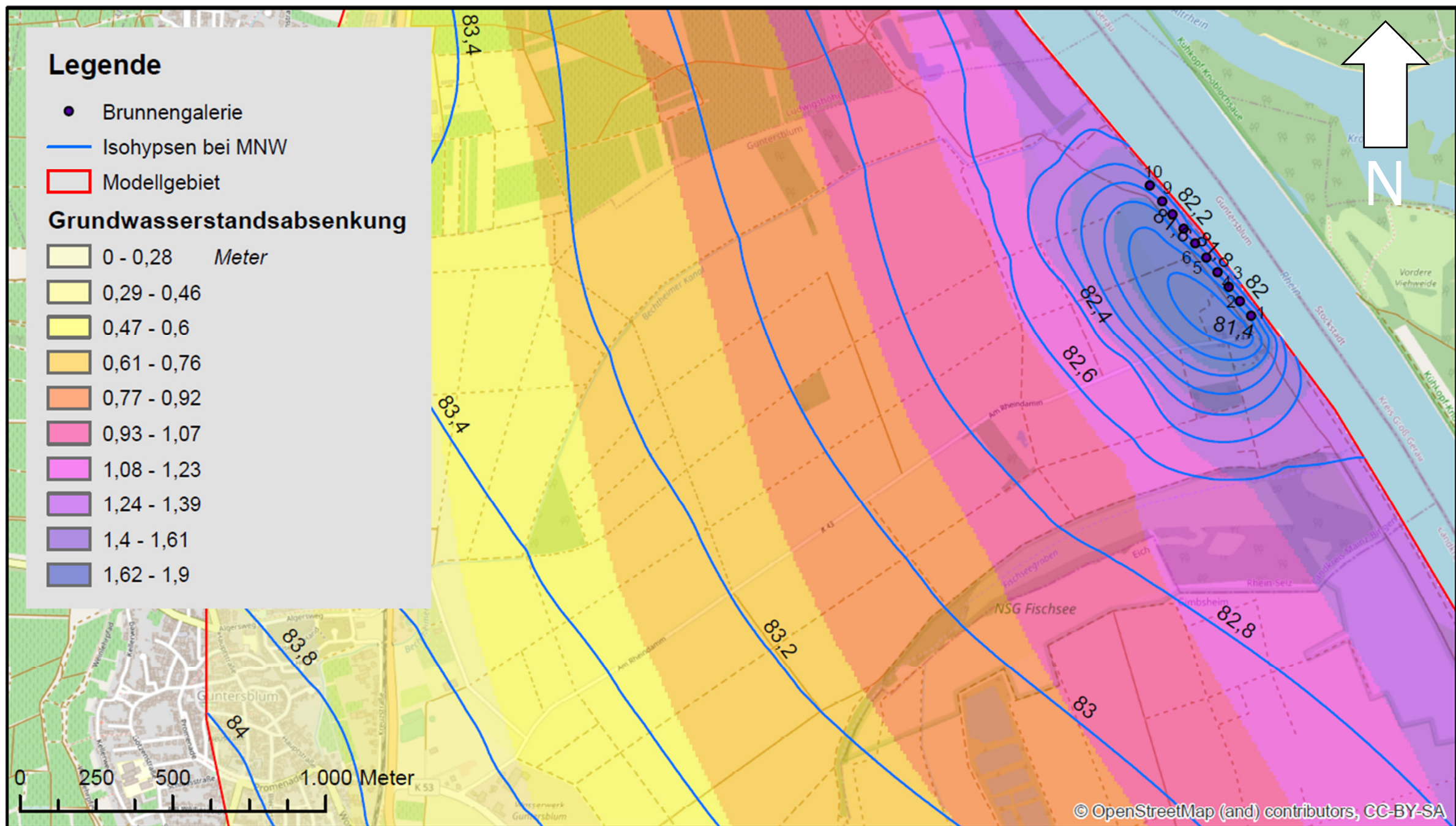
Abb. 5: Grundwassermodell Guntersblum.
