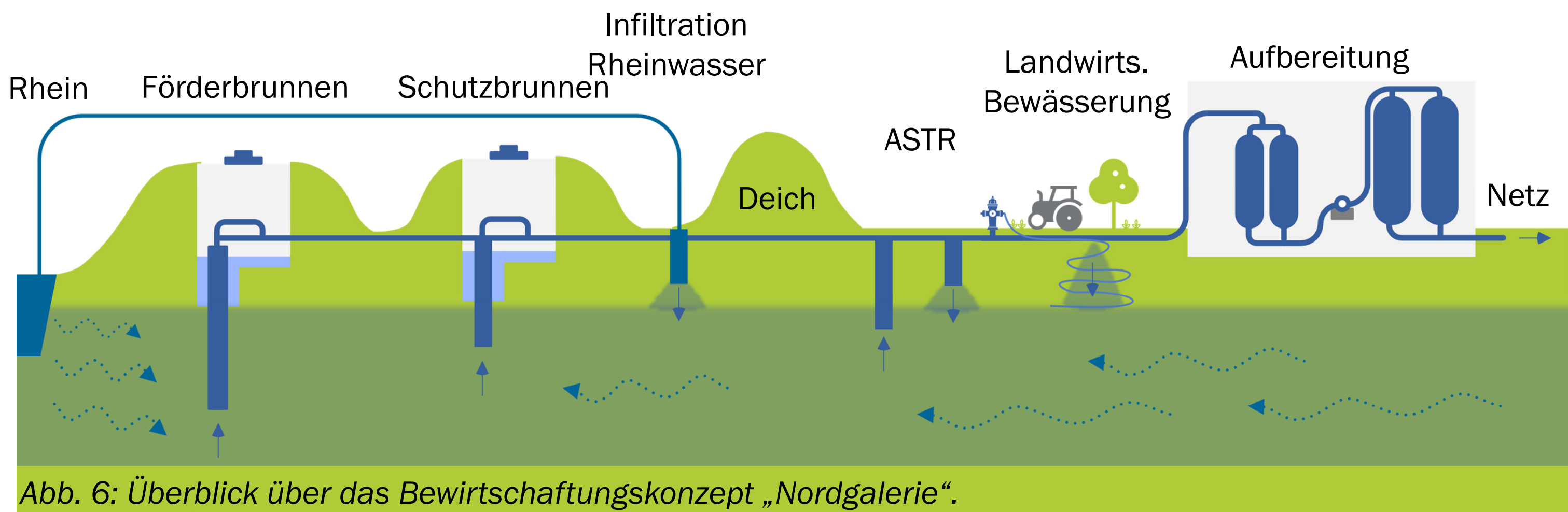
Abb. 6: Überblick über das Bewirtschaftungskonzept „Nordgalerie“.
