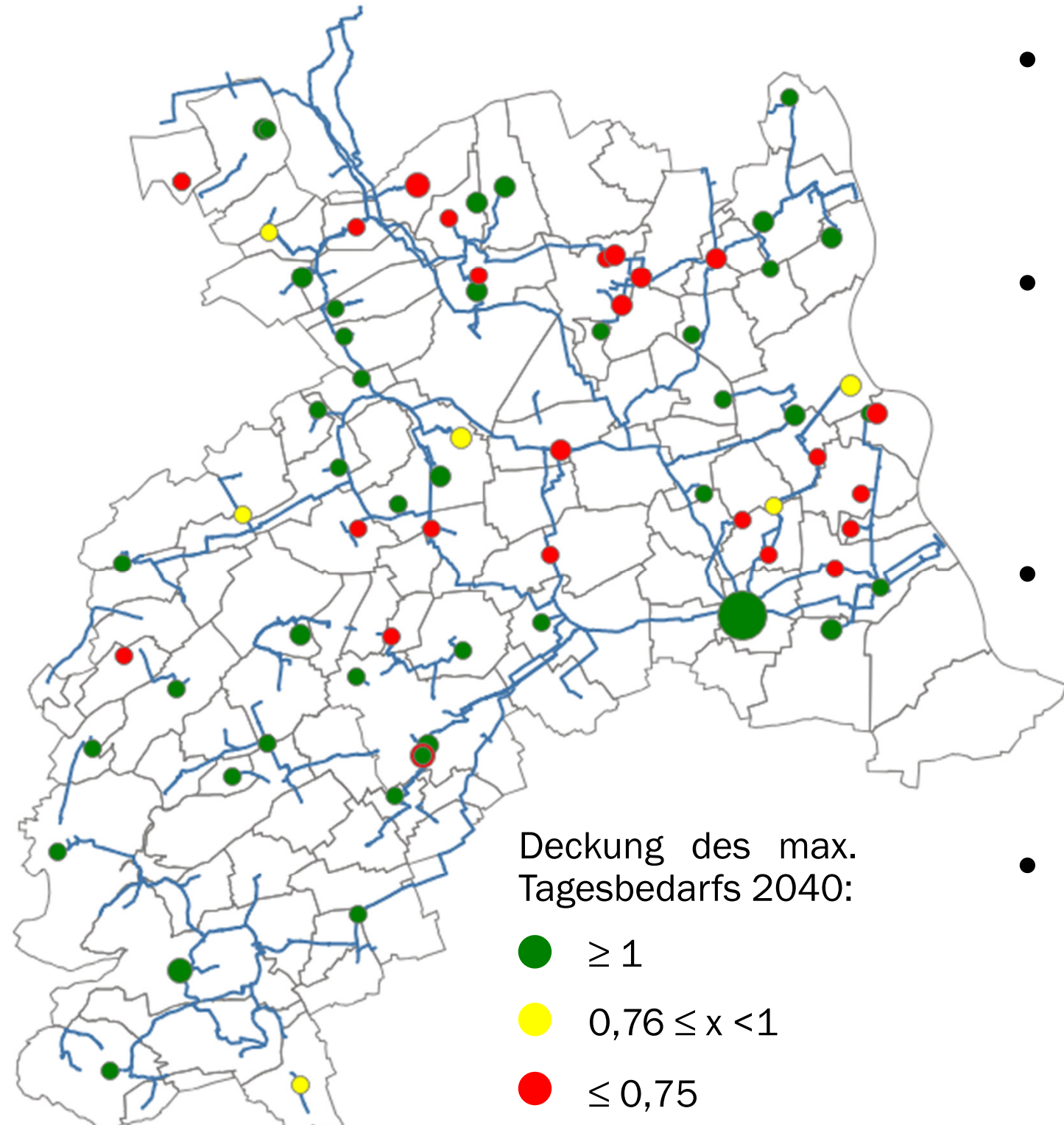
Abb. 3: Klassifizierung von Vulnerabilitäten im Versorgungsgebiet.
